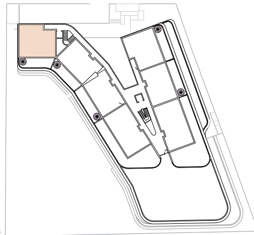
PLANTA TERCERA
